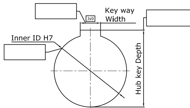
Hub key Deetail Keyway to DIN 6885-P1
